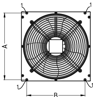
Рис. 5. Межосевое расстояние крепления скоб
