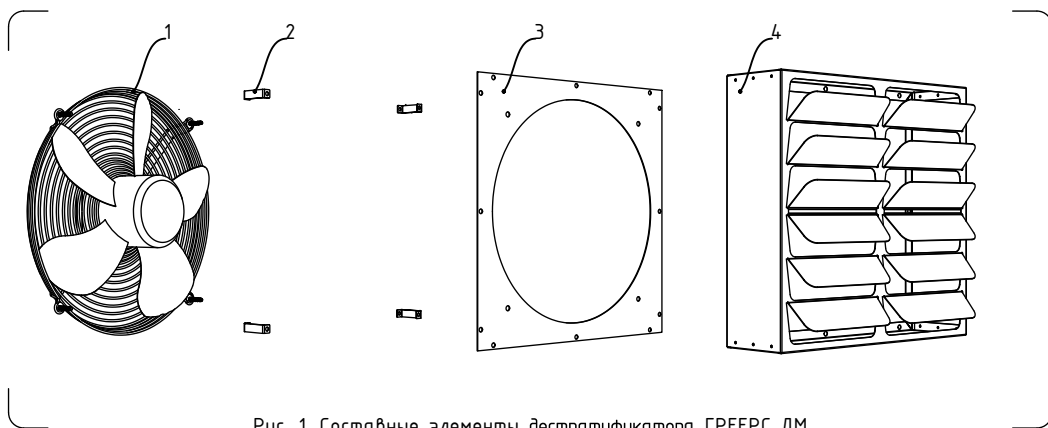
Рис. 1. Составные элементы дестратификатора ГРЕЕРС ДМ
