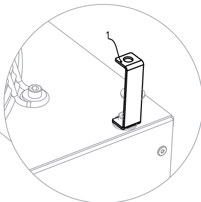
Рис. 4. Крепление монтажной шпильки с помощью скоб
