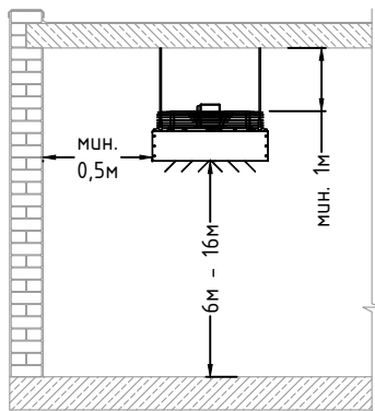
Рис. 3. Рекомендуемые расстояния при монтаже монтаже 3-го и 4-го типоразмера
