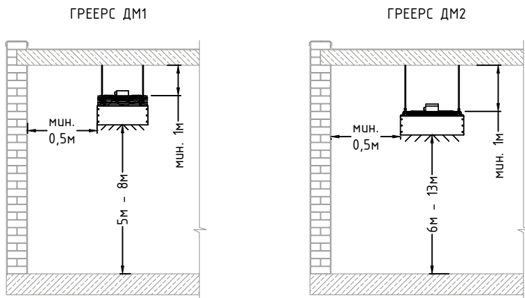
Рис. 2. Рекомендуемые расстояния при монтаже дестратификаторов 1-го и 2-го типоразмера
