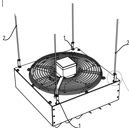
Рис. 4. Крепление монтажной шпильки с помощью скоб
