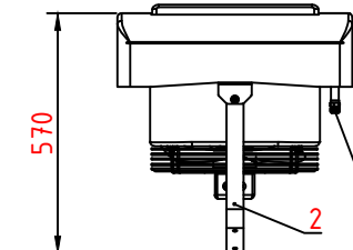
Вид сверху
