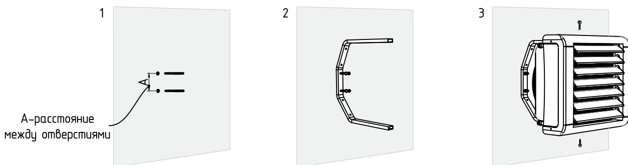
Рис. 5. Монтаж консоли
