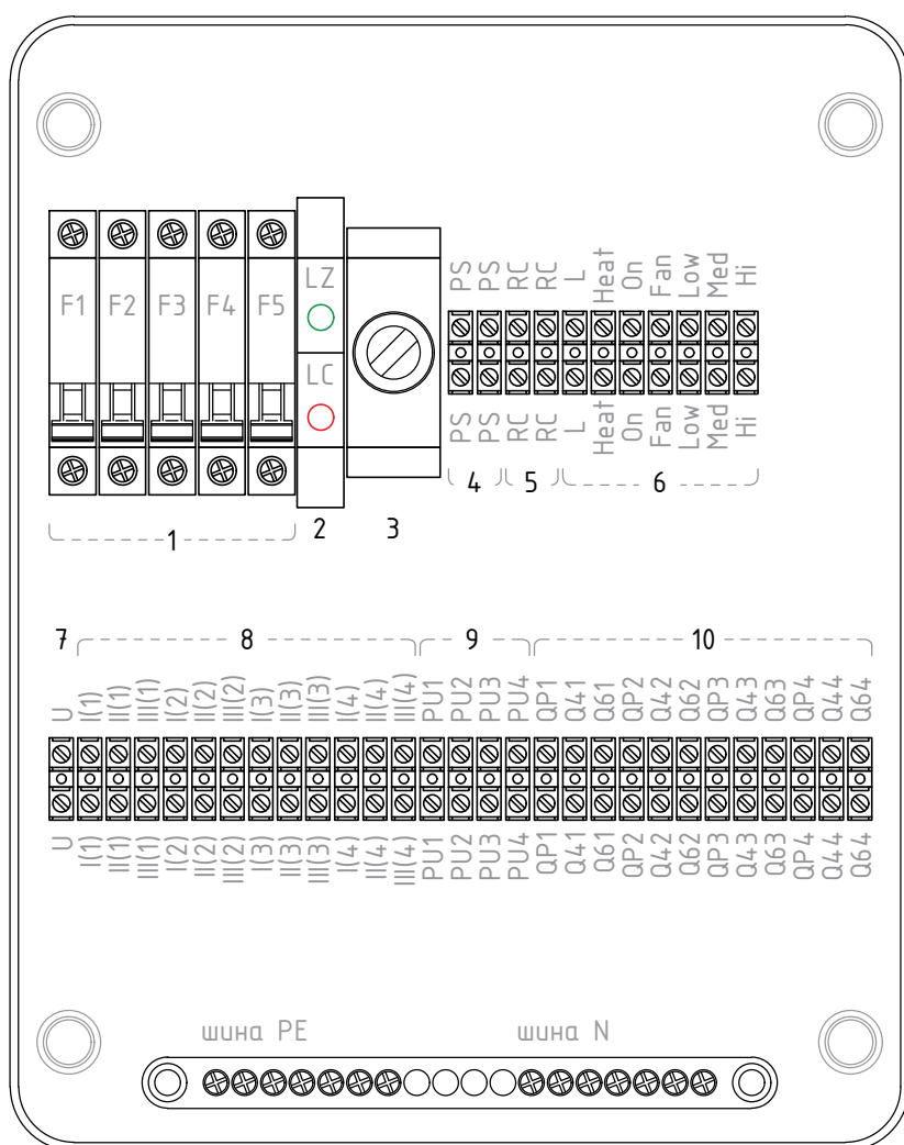
Рис. 2. Схема расположения клемм в БПУ-У для подключения оборудования
