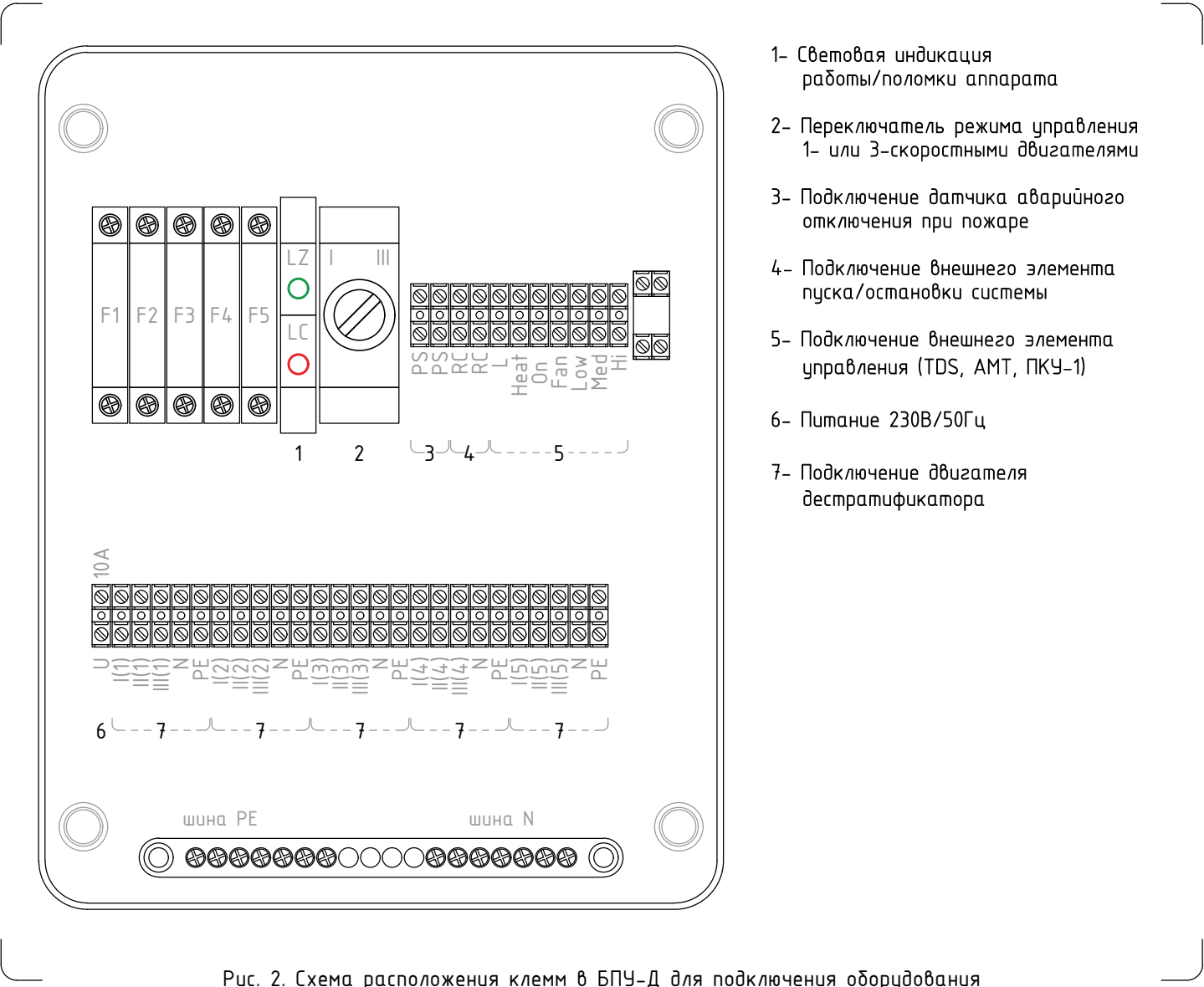
Рис. 2. Схема расположения клемм в БПУ-Д для подключения оборудования
