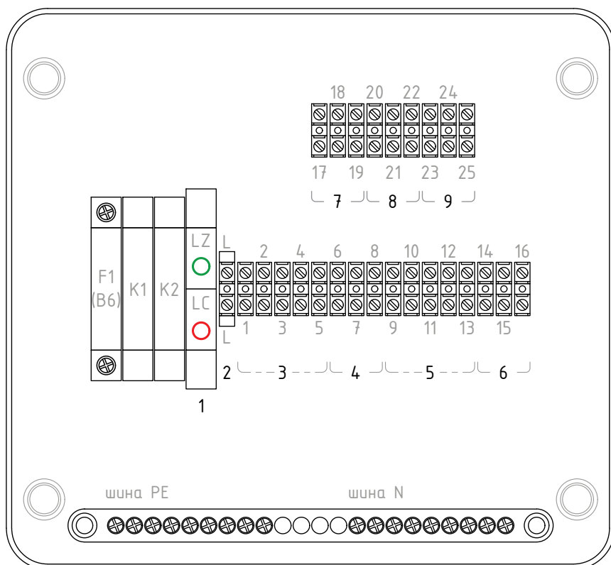
Рис. 2. Схема расположения клемм в БПУ-КС для подключения дополнительного оборудования
