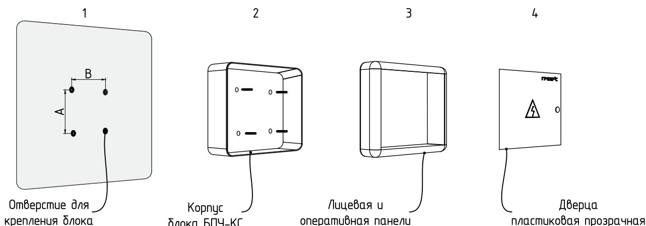
Рис. 1. Порядок монтажа блока на стене
