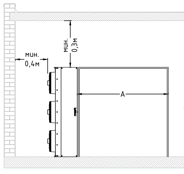
Установка воздушной завесы ЗВП-М сбоку от проема
