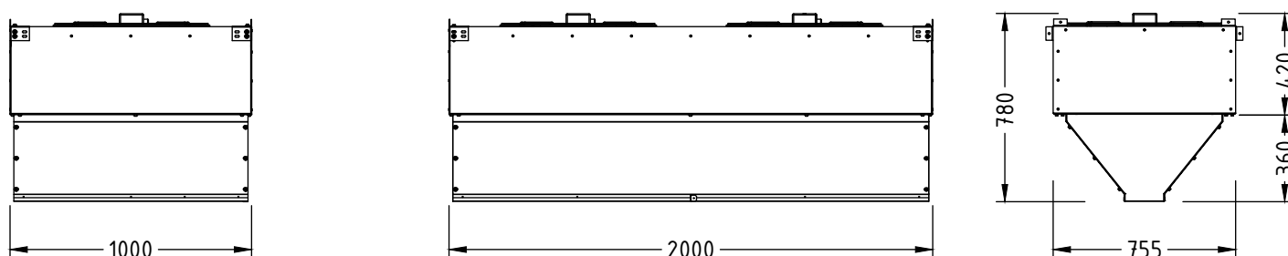
ГРЕЕРС ЗВП-М4-100 | 200
