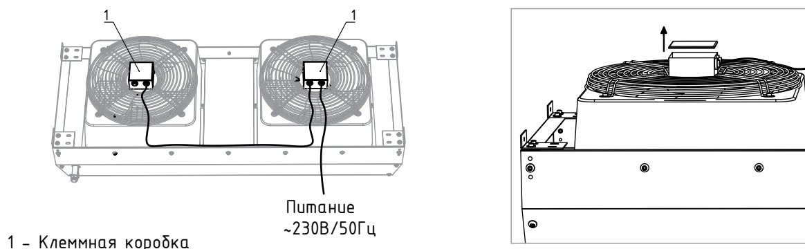
Рис. 7. Порядок подключения электропитания воздушной завесы серии ЗВП-М-Н/В
