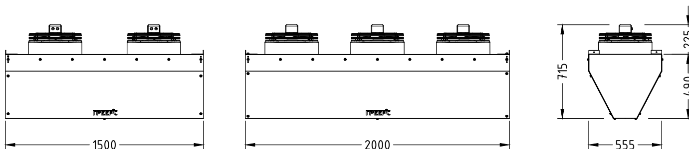
ГРЕЕРС ЗВП-М1-150 | 200
