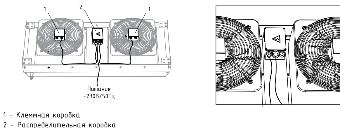
Рис. 8. Порядок подключения электропитания воздушной завесы серии ЗВП-М-Е
