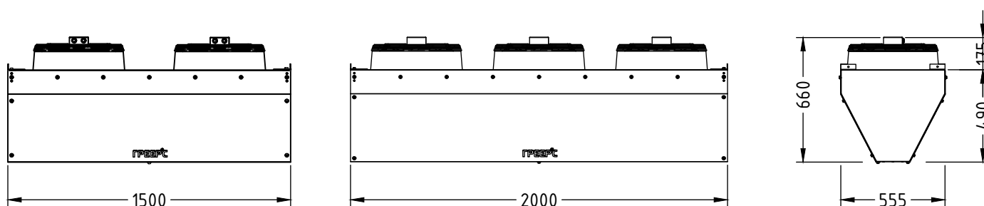
ГРЕЕРС ЗВП-М2-150 | 200
