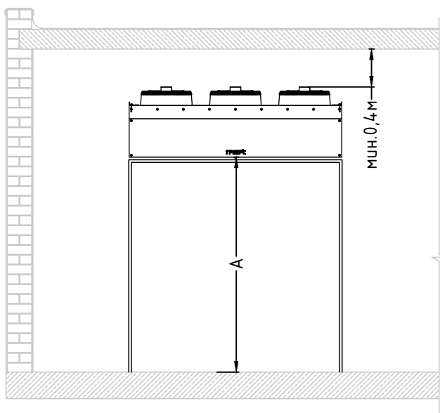
Установка воздушной завесы ЗВП-М над проемом
