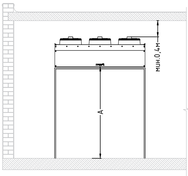
Установка воздушной завесы ЗВП-М над проемом
