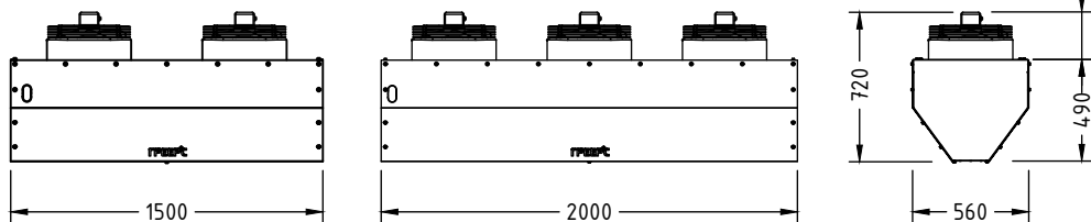
ГРЕЕРС ЗВП-М2-150 | 200
