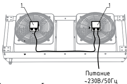
1 – Клеммная коробка
