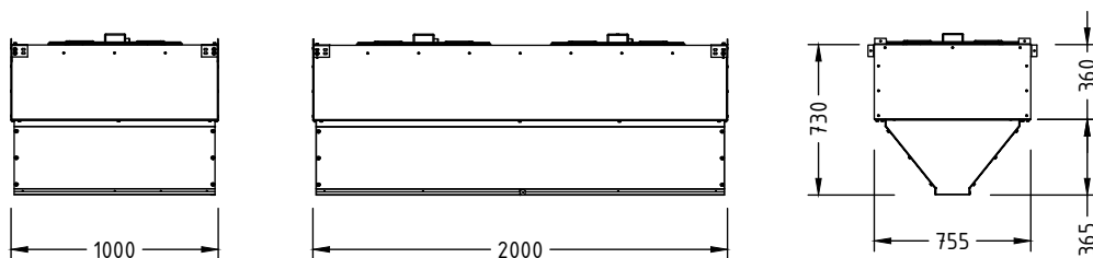
ГРЕЕРС ЗВП-М4-100 | 200
