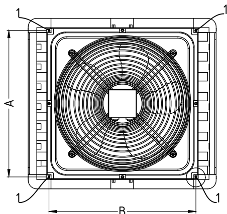
Рис. 5. Межсоедовое расстояние крепления скоды
