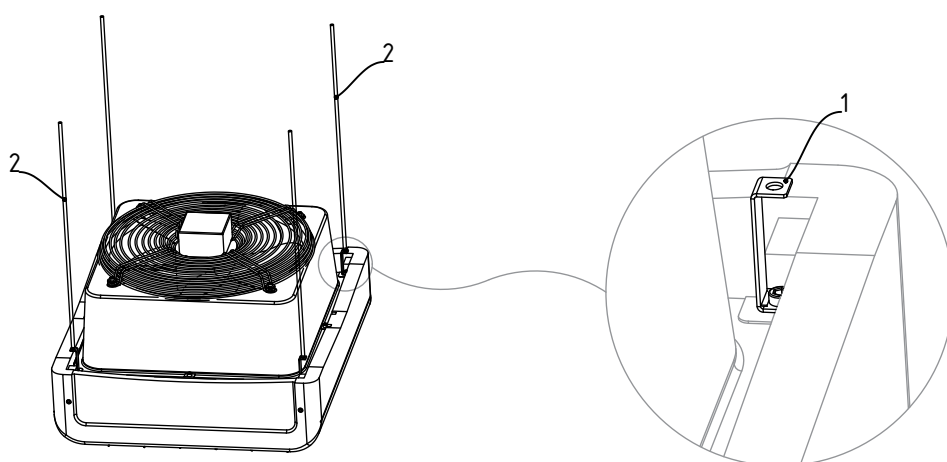
Рис. 4. Крепление монтажной шпильки с помощью скоб
