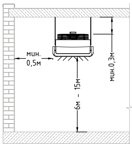
Рис. 3. Рекомендуемые расстояния при монтаже 3-го и 4-го типоразмера
