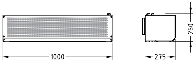
ГРЕЕРС ЗВ-Б2-100Е
