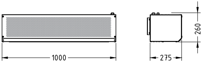
ГРЕЕРС ЗВ-Б2-100Н
