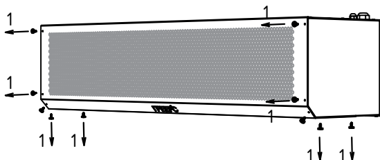
1. Снятие винтов
