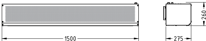
ГРЕЕРС ЗВ-Б2-150Е
