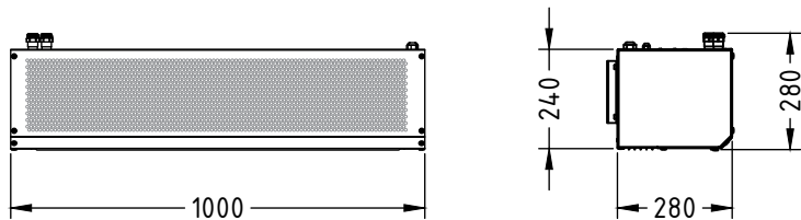
ГРЕЕРС ЗВ-Б2-100В
