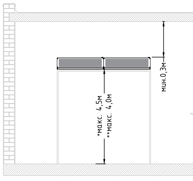
Установка воздушных завес ЗВ-Б2 над проемом
