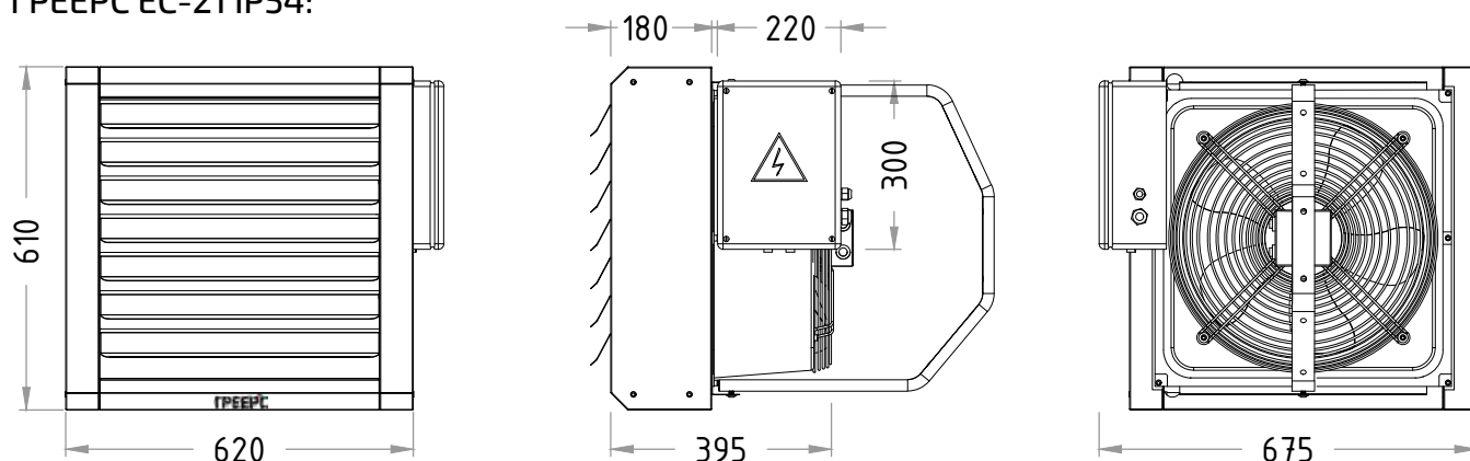
ГРЕЕРС ЕС-21 IP54:
