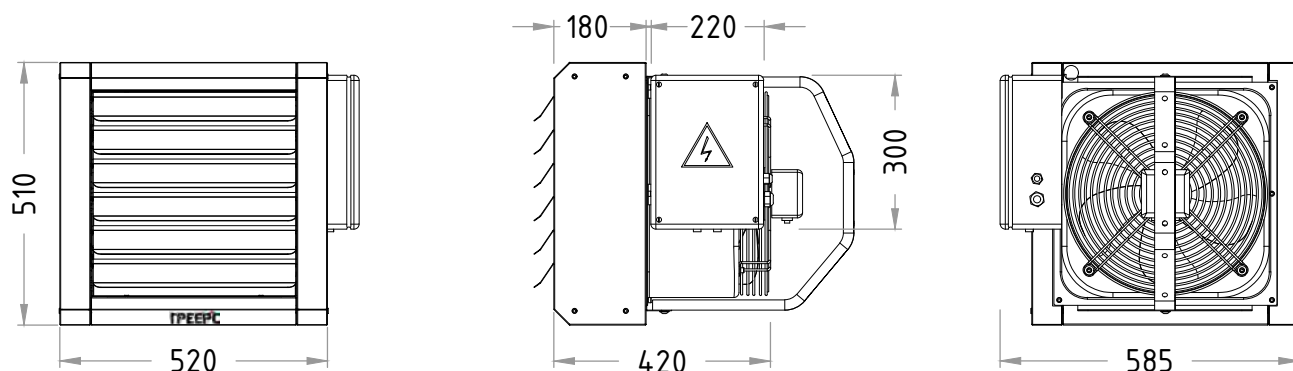
ГРЕЕРС ЕС-21 IP54:
