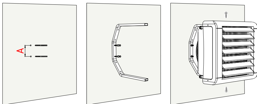
Рис. 4. Монтаж консоли
