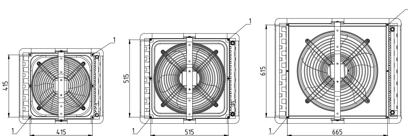
Рис. 3. Расстояния между крепежными держателями
