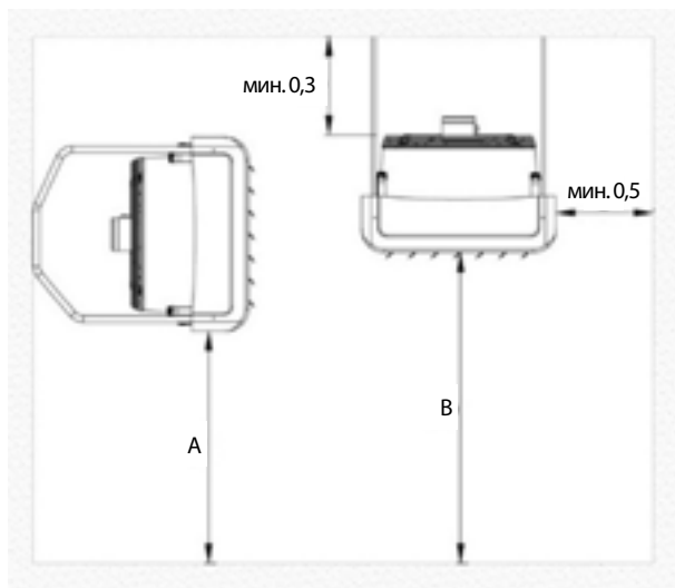
Рис. 2. Рекомендуемые расстояния для монтажа
