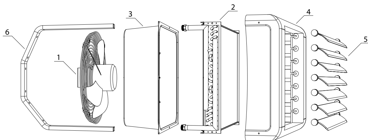
Рис. 1. Составные элементы тепловентилятора ГРЕЕРС ВС
