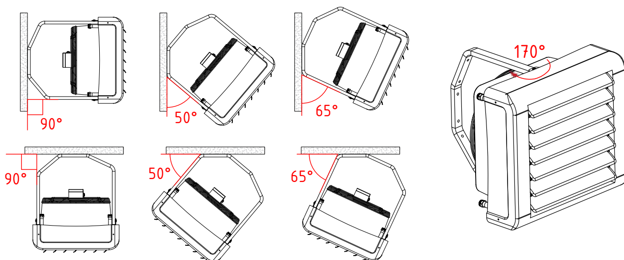
Рис. 5. Варианты установки монтажной консоли
