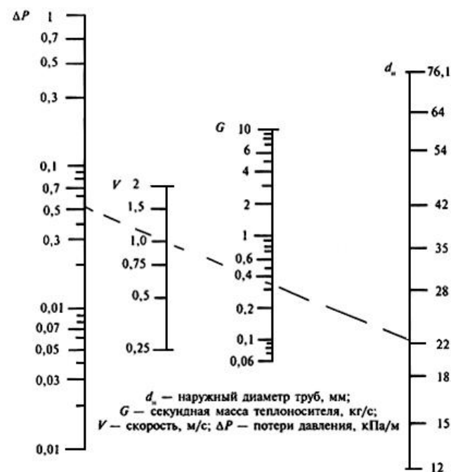
Рисунок В.2 - Система отопления
