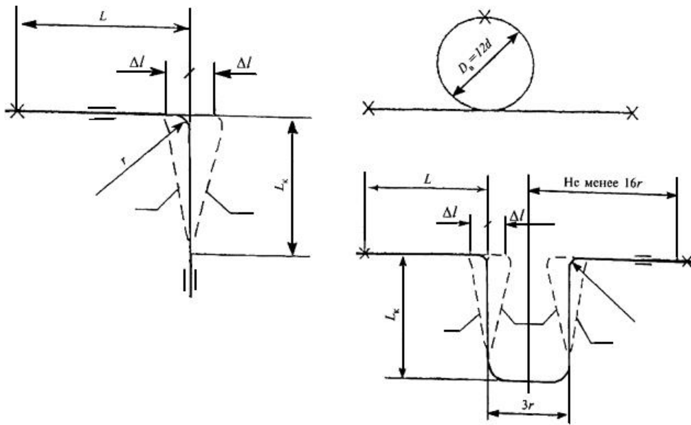
Рисунок Д.1 - Расчетные схемы гнутых компенсаторов*
