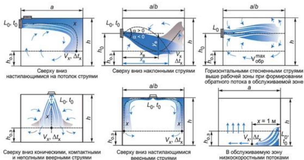
Рисунок Ж.1 - Основные схемы подачи приточного воздуха
